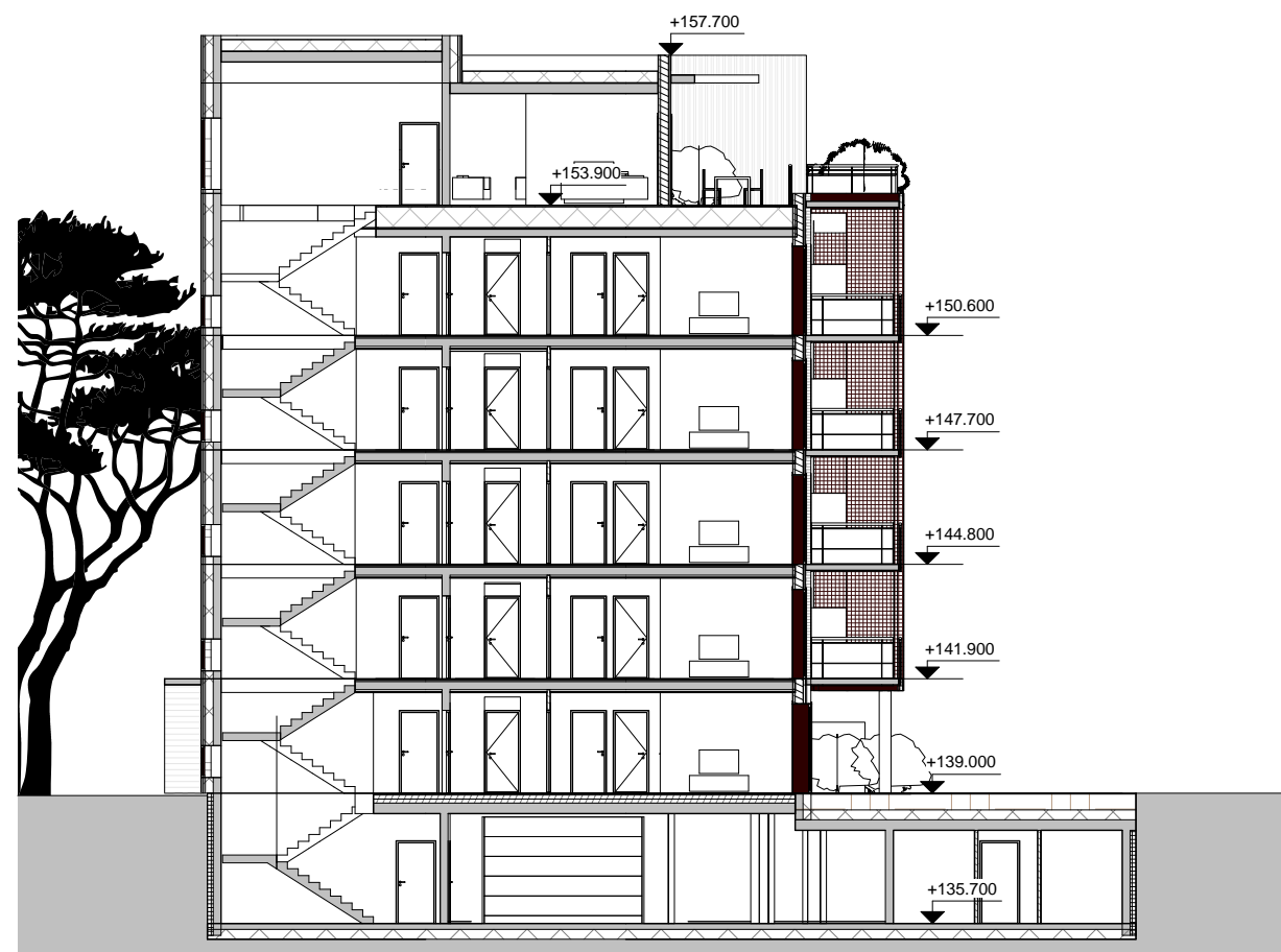
Snitt Bygg 1
