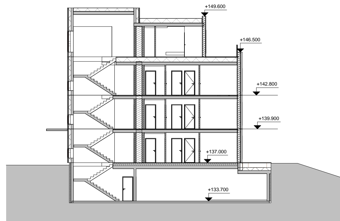
Snitt Bygg 3
