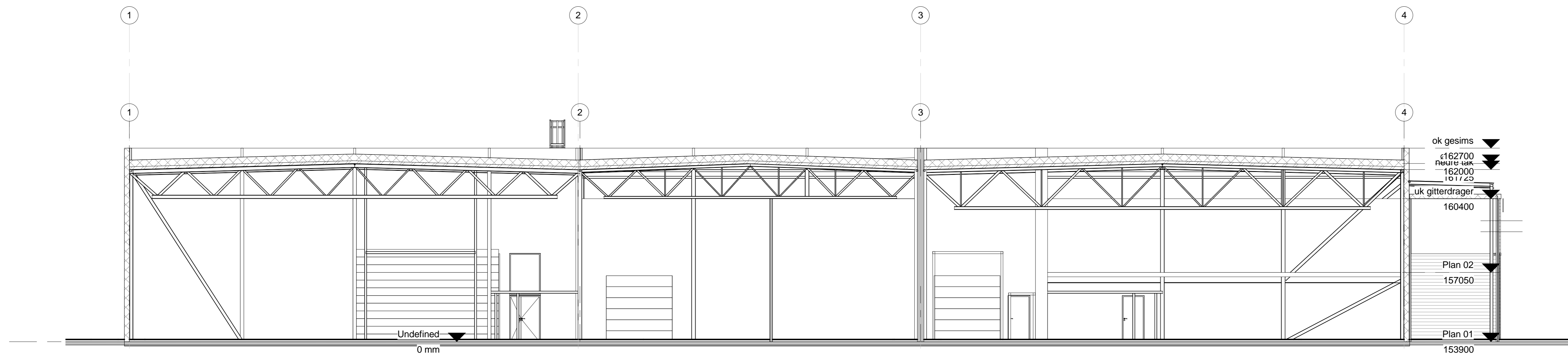
2 Snitt B-B 1 : 100
