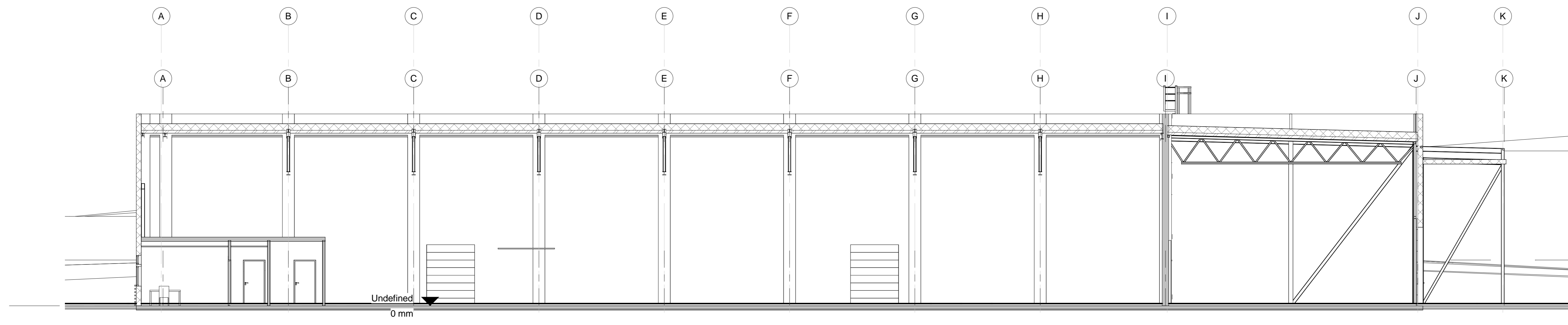
1 Snitt A-A 1 : 100
