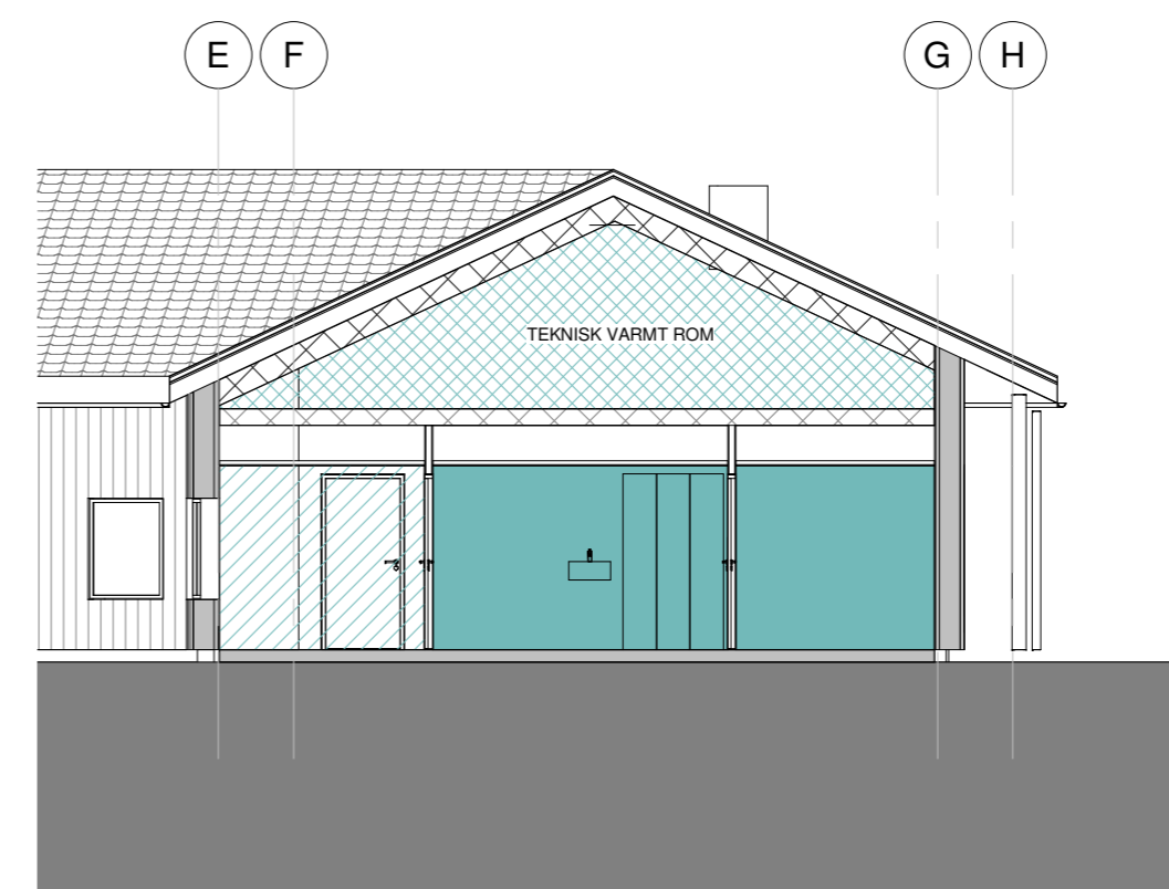
3 CC 1 : 100
