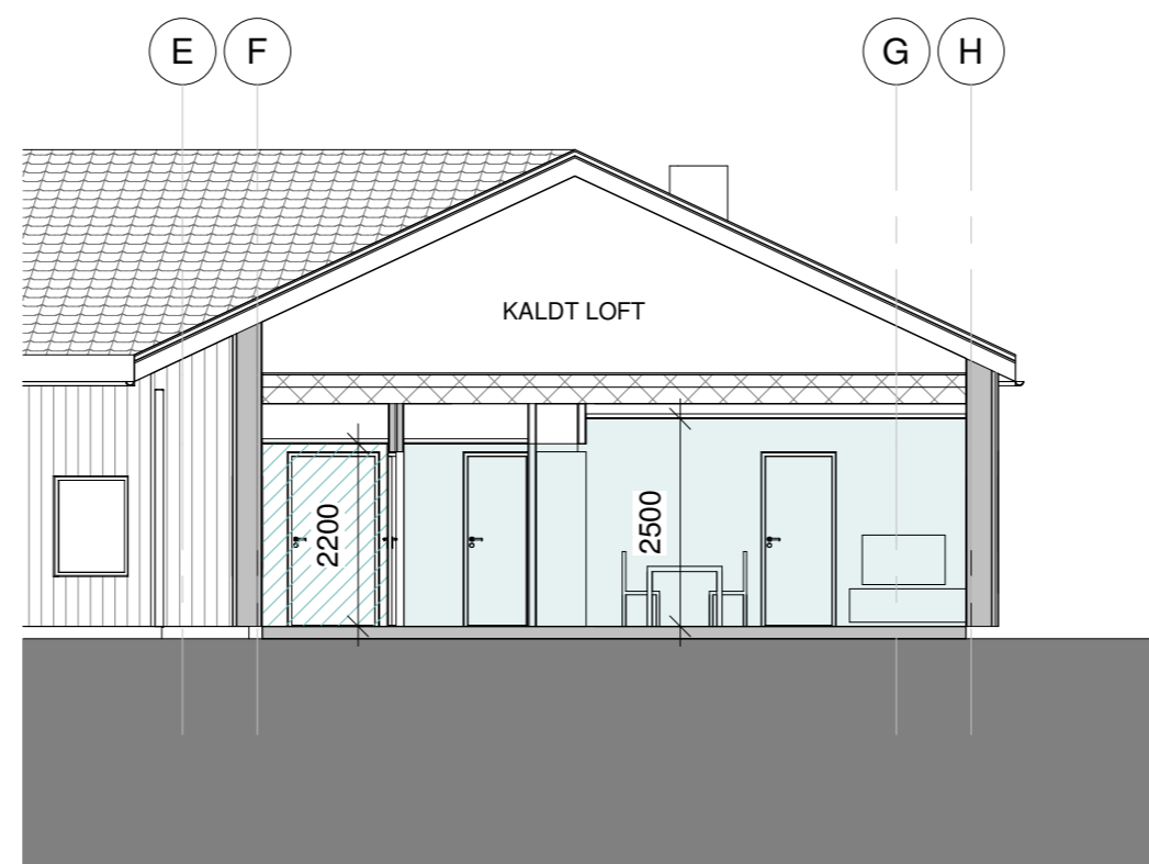
2 BB 1 : 100
