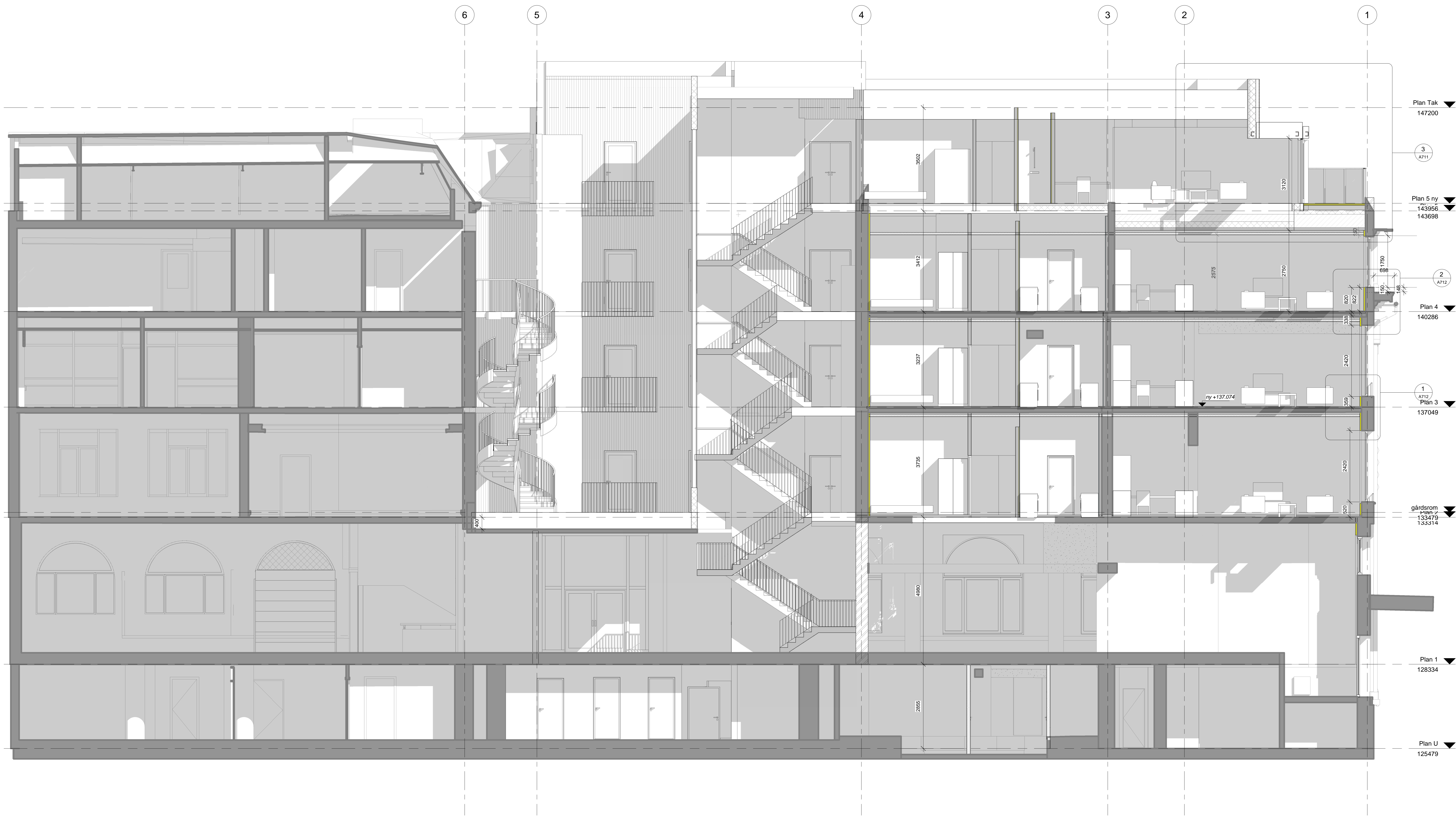
1 Snitt 1 1 : 50
