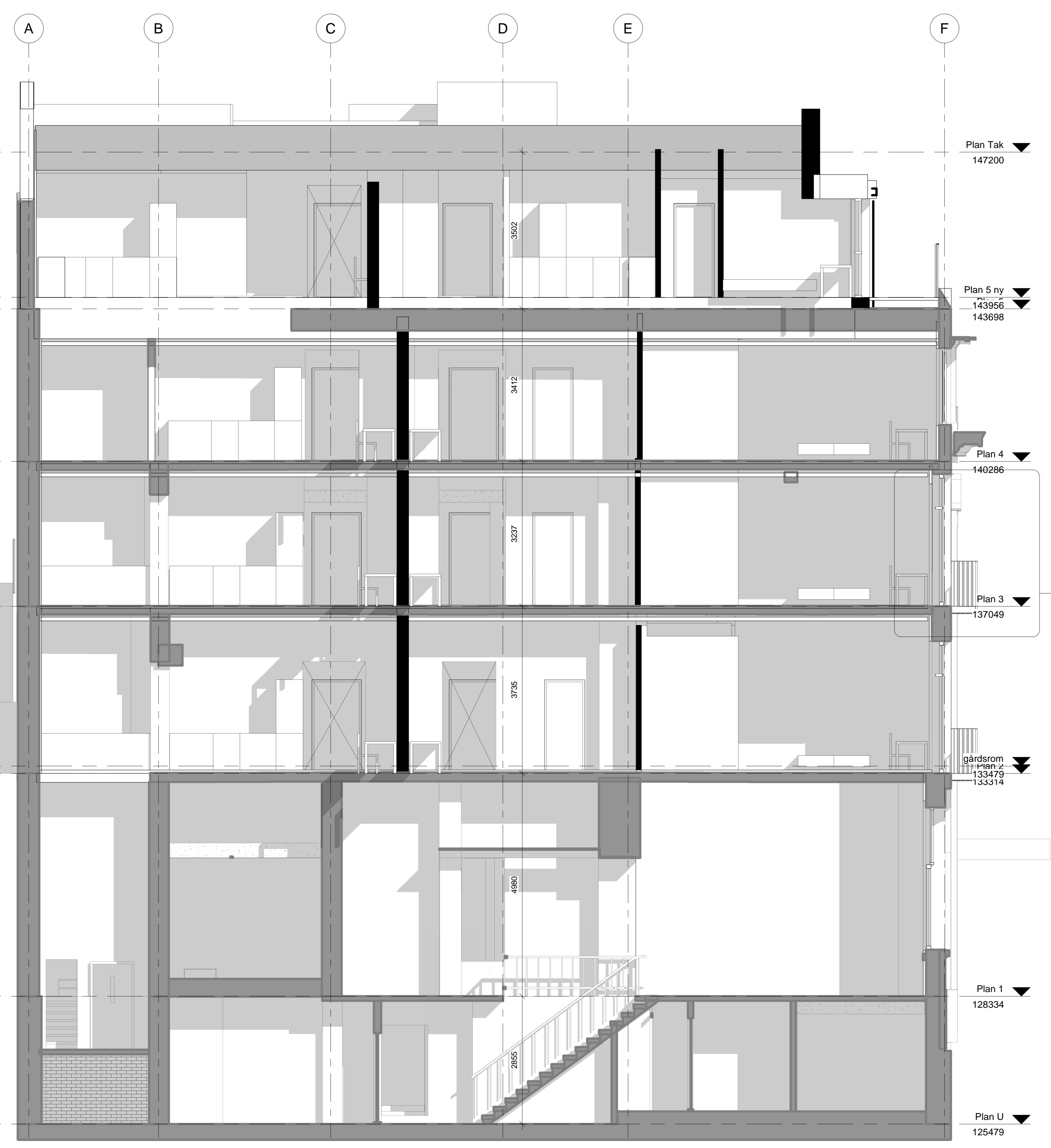
7 Snitt 3 1 : 50
